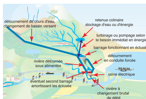
"Illustration 7" Schéma d'un barrage à conduite forcée CRCK du Centre
