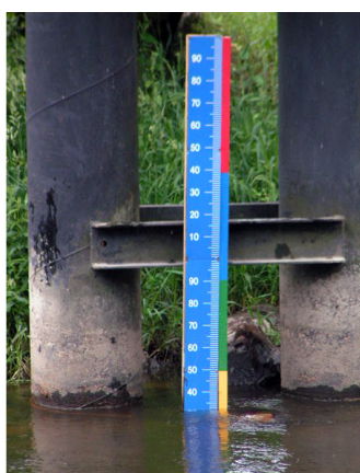
"Illustration 15" Limnimètre - Eric Chazal KCM
